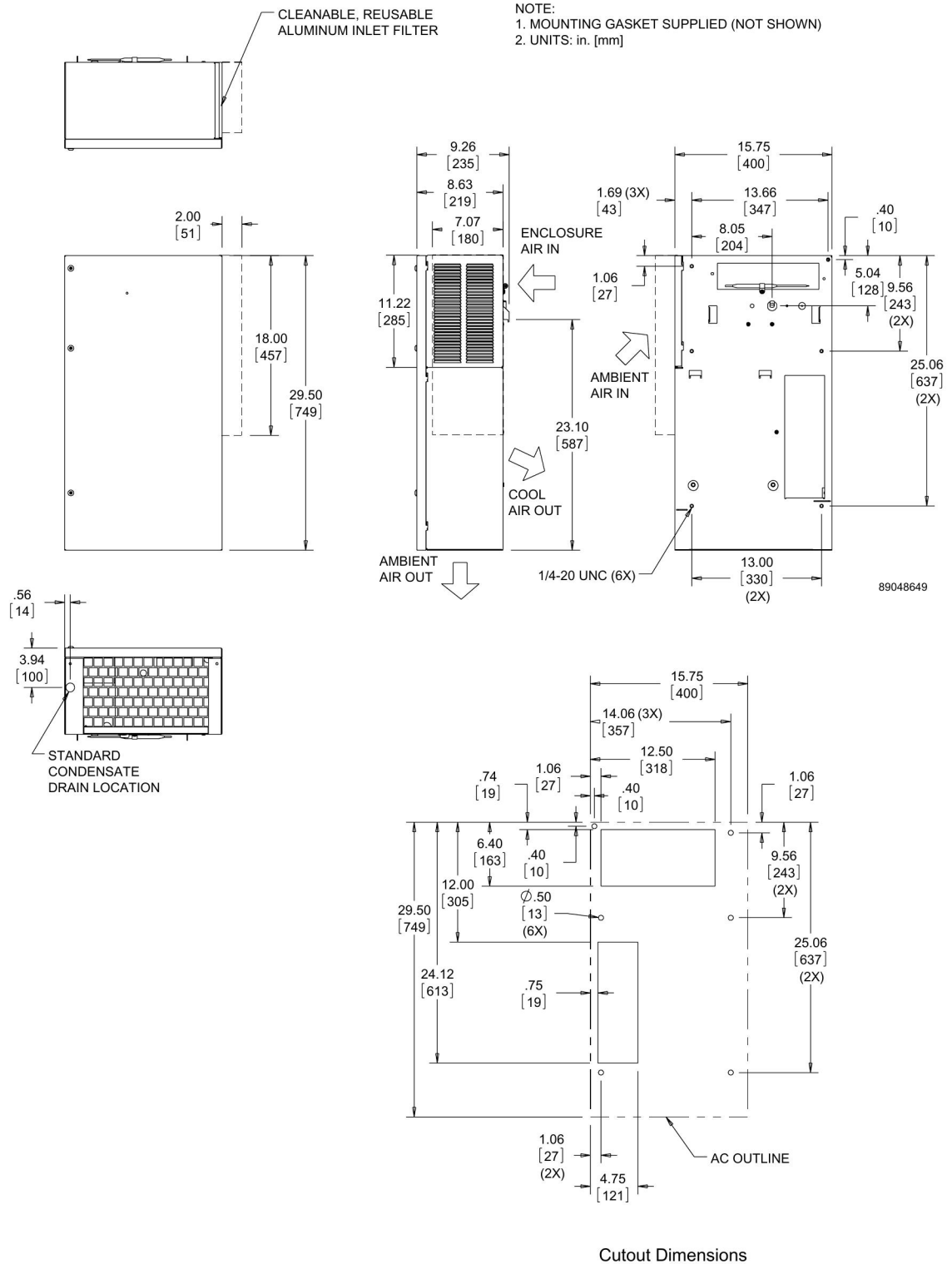
Cutout Dimensions
